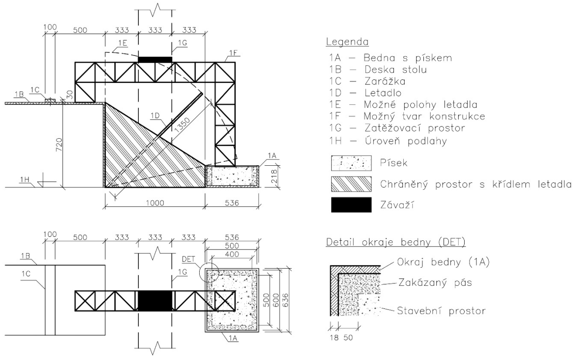
Obr. 1 - Schéma konstrukce
